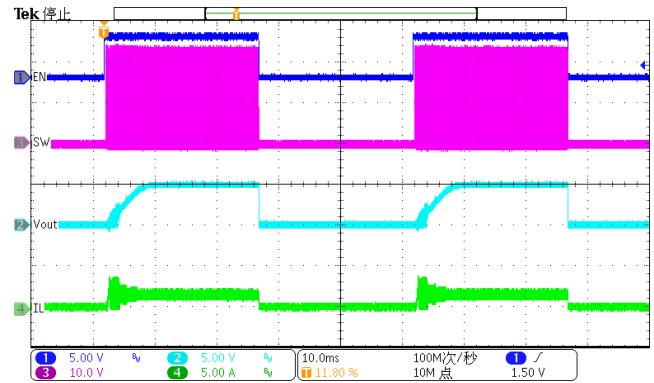
Figure 14. EN toggle ( I_{LOAD}=1.5A )
