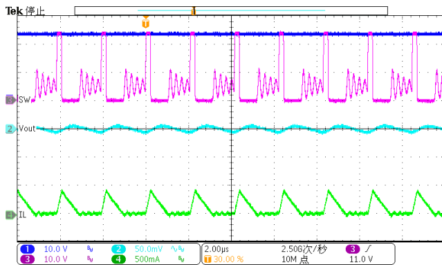
Figure 19. Output Ripple (ILOAD=0.1mA)
