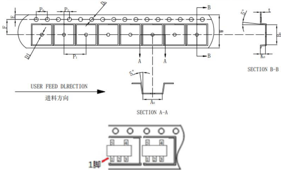
SOT23-5
