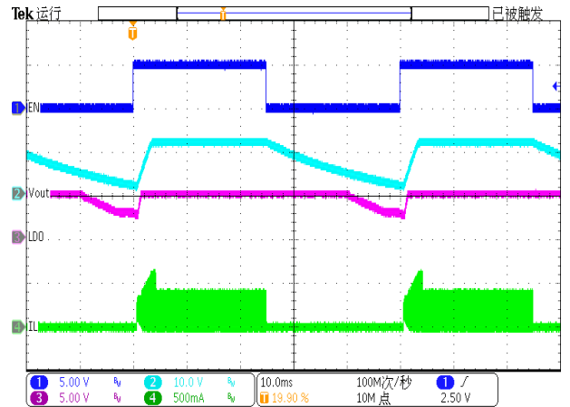
Figure 20. EN toggle (Iload=10mA)
