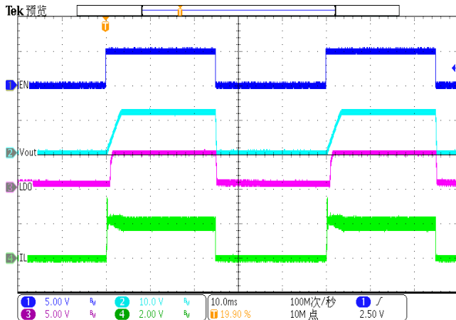
Figure 19. EN toggle (Iload=2A)
