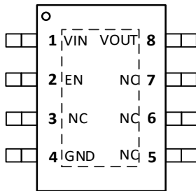
SCT71403FxxQMTER EMSOP3x3-8 Package
