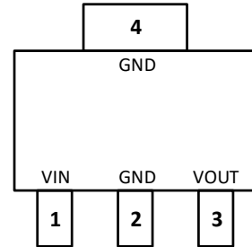
SCT71403FxxQTXER SOT223-4 Package
