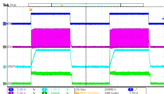
Figure 15. EN toggle (Iload=0.1A)
