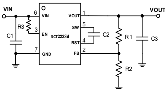
4.2V-8.5V, Synchronous Buck Converter Module
