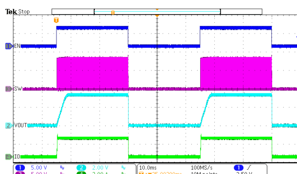
Figure 16. EN toggle (Iload=2A)
