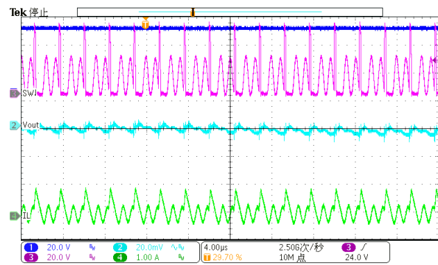
Figure 37. Output Ripple, DCM (Iload=100mA)
