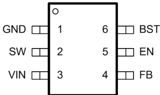
TSOT23-6 Top View (2.8mm x 2.8mm)
