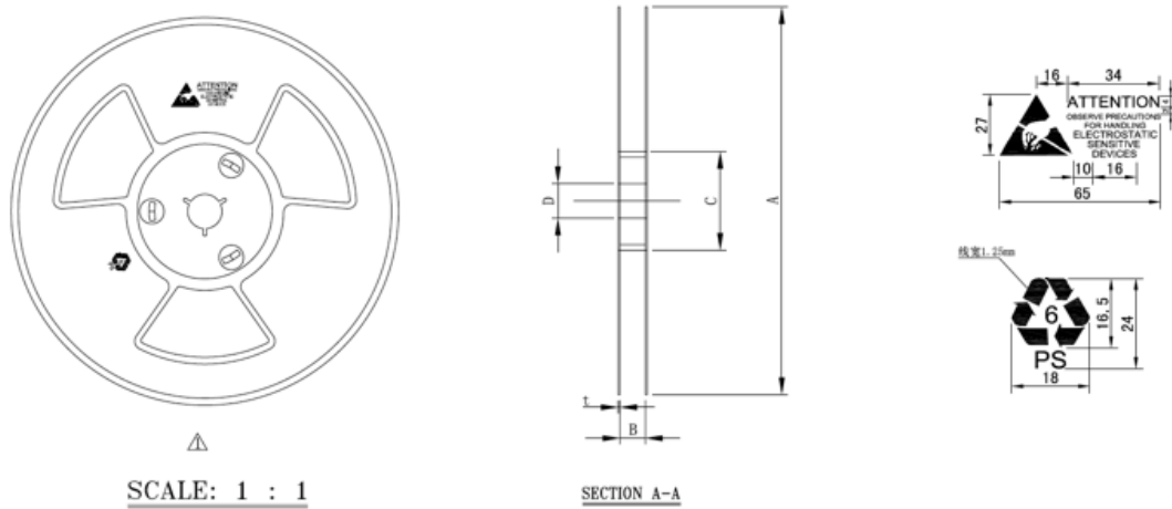
REEL DIMENSIONS
