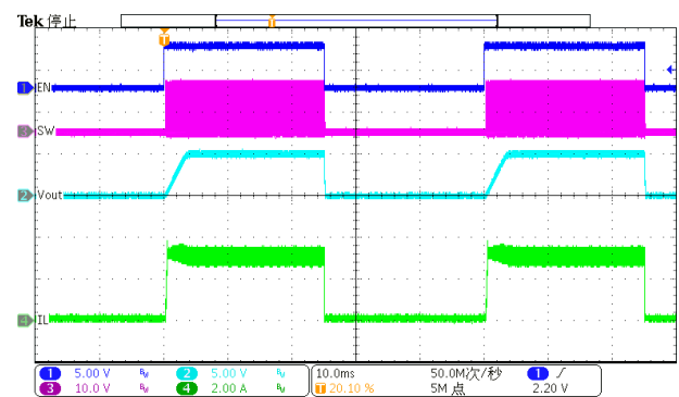
Figure 15. EN toggle ( I_{LOAD}=3A )
