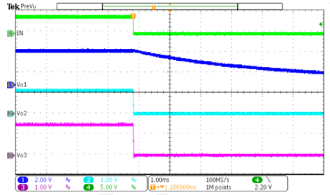
Figure 11. EN Off
