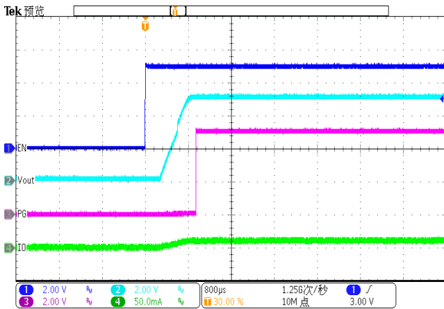
Figure 46. Enable (Iload=10mA)
