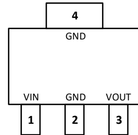
SCT71403FxxQTXER SOT223-4L Package
