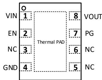
SCT71403FxxQDTBR TQFN3X3-8L Package
