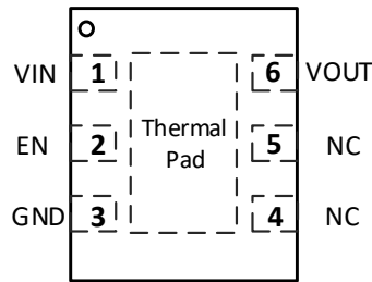
SCT71403FxxQDVAR TQFN2X2-6L Package
