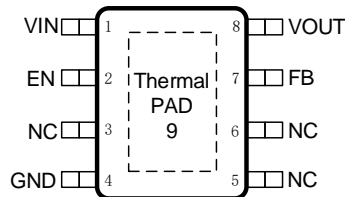
SCT71403A05QMTER EMSOP-8L Package
