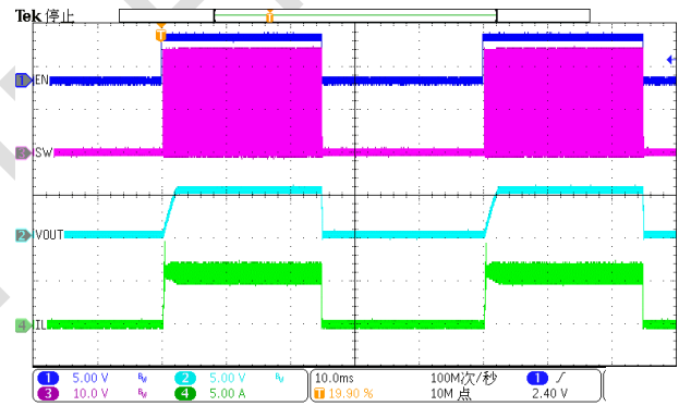
Figure 16. EN toggle (Iload=6A)
