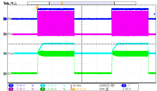
Figure 22. EN toggle ( I_{LOAD}=10A )
