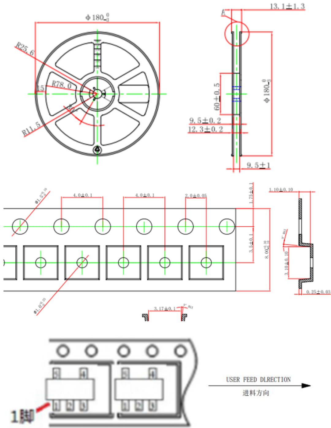
SOT23-5L
