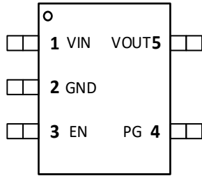
SCT71005FxxQTWDR SOT23-5L Package
