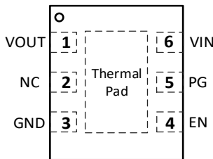
SCT71005FxxQDVAR DFN2X2-6L Package
