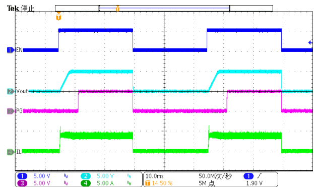
Figure 16. EN toggle (Iload=4A)
