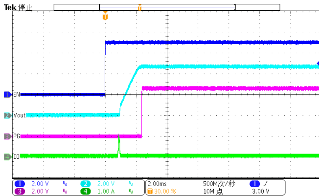
Figure 41. Enable (Iload=10mA)
