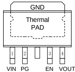
SCT71405FxxAQOWCR TO252-4L Package
