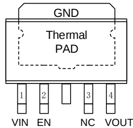
SCT71405FxxQOWCR TO252-4L Package
