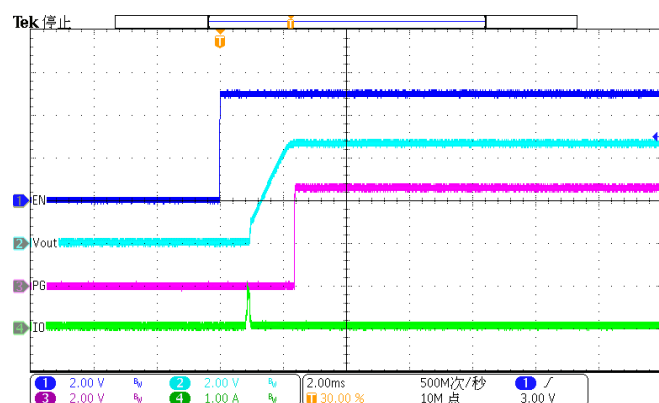
Figure 41. Enable (Iload=10mA)
