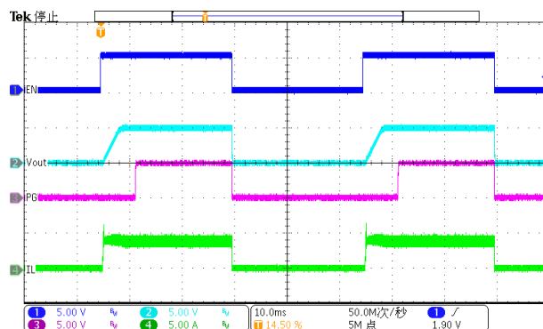
Figure 16. EN toggle (Iload=4A)
