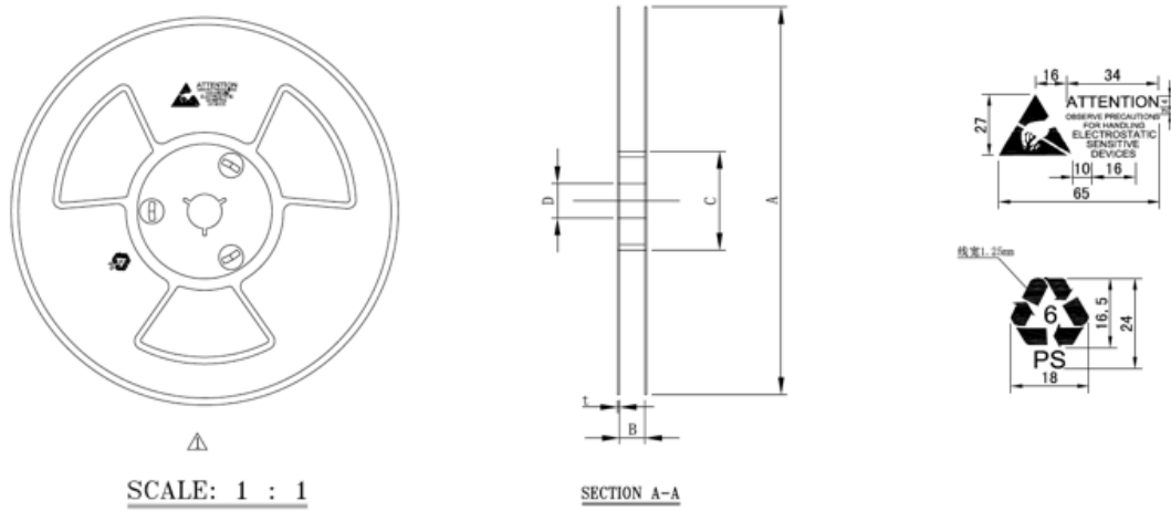
REEL DIMENSIONS
