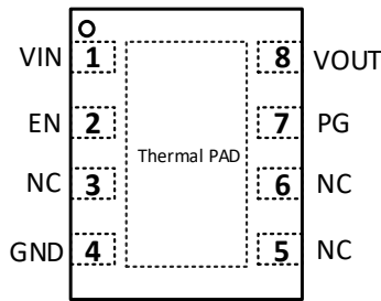
SCT71403FxxQDTBR DFN3X3-8L Package
