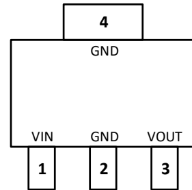
SCT71403FxxQTXER SOT223-4L Package
