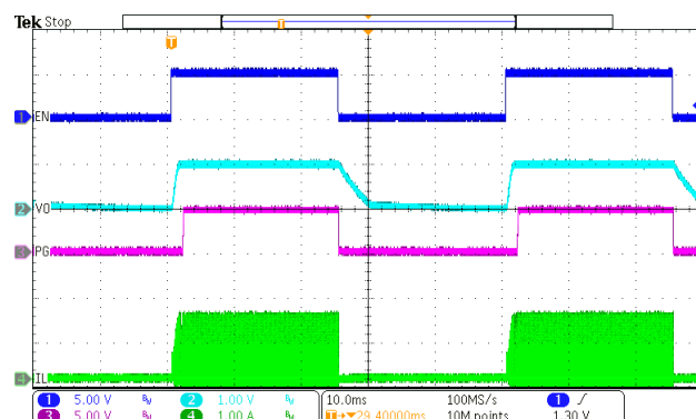
Figure 14. EN toggle PFM (Iload=10mA)
