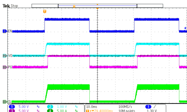
Figure 13. EN toggle (Iload=6A)
