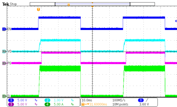
Figure 13. EN toggle (Iload=12A)
