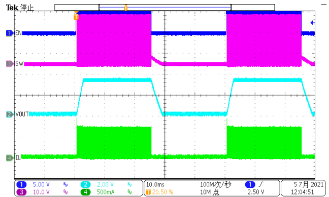
Figure 17. EN toggle (Iload=0.1A)
