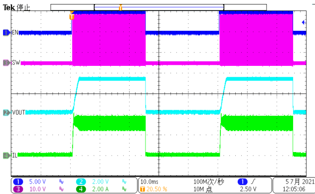
Figure 16. EN toggle (Iload=3A)
